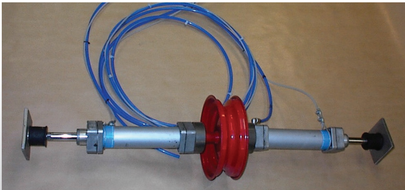
Slanghållare med två pneumatiskt styrda kolvar som låser fast slanghållaren i korrekt position
